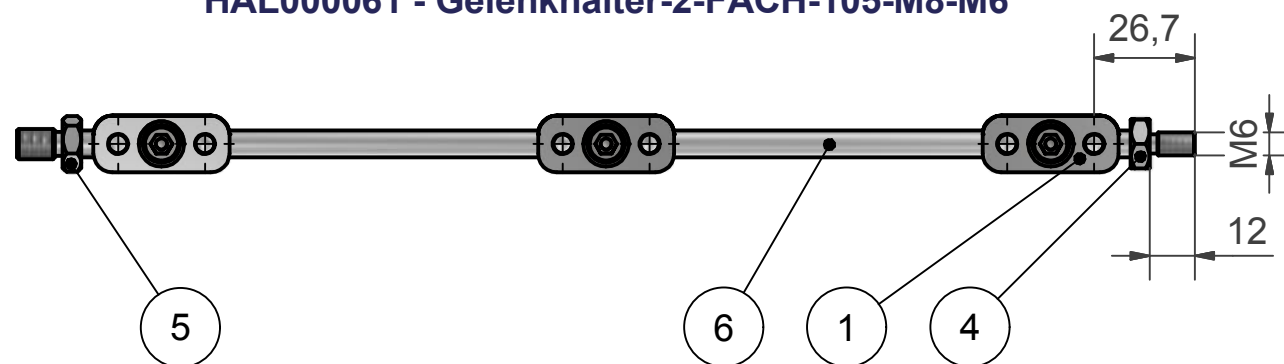
HAL000061 - Gelenkhalter-2-FACH-105-M8-M6
