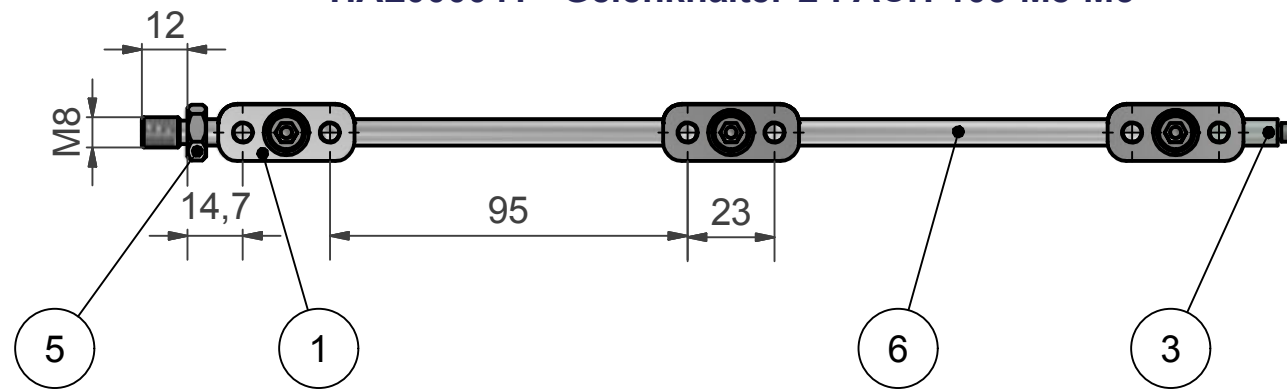
HAL000041 - Gelenkhalter-2-FACH-105-M8-M5
